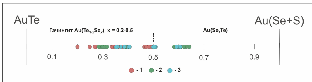
Рис. 3. Химический состав халькогенидной части гачингита и его Se-доминантного аналога, выраженный отношением (Se+S)/(Te+S+Se). 1 – рудопоявление Гачинг из [Tolstykh et al., 2022], 2 – рудопоявление Гачинг из [Tolstykh et al., 20231], 3 – Озерновское месторождение.
