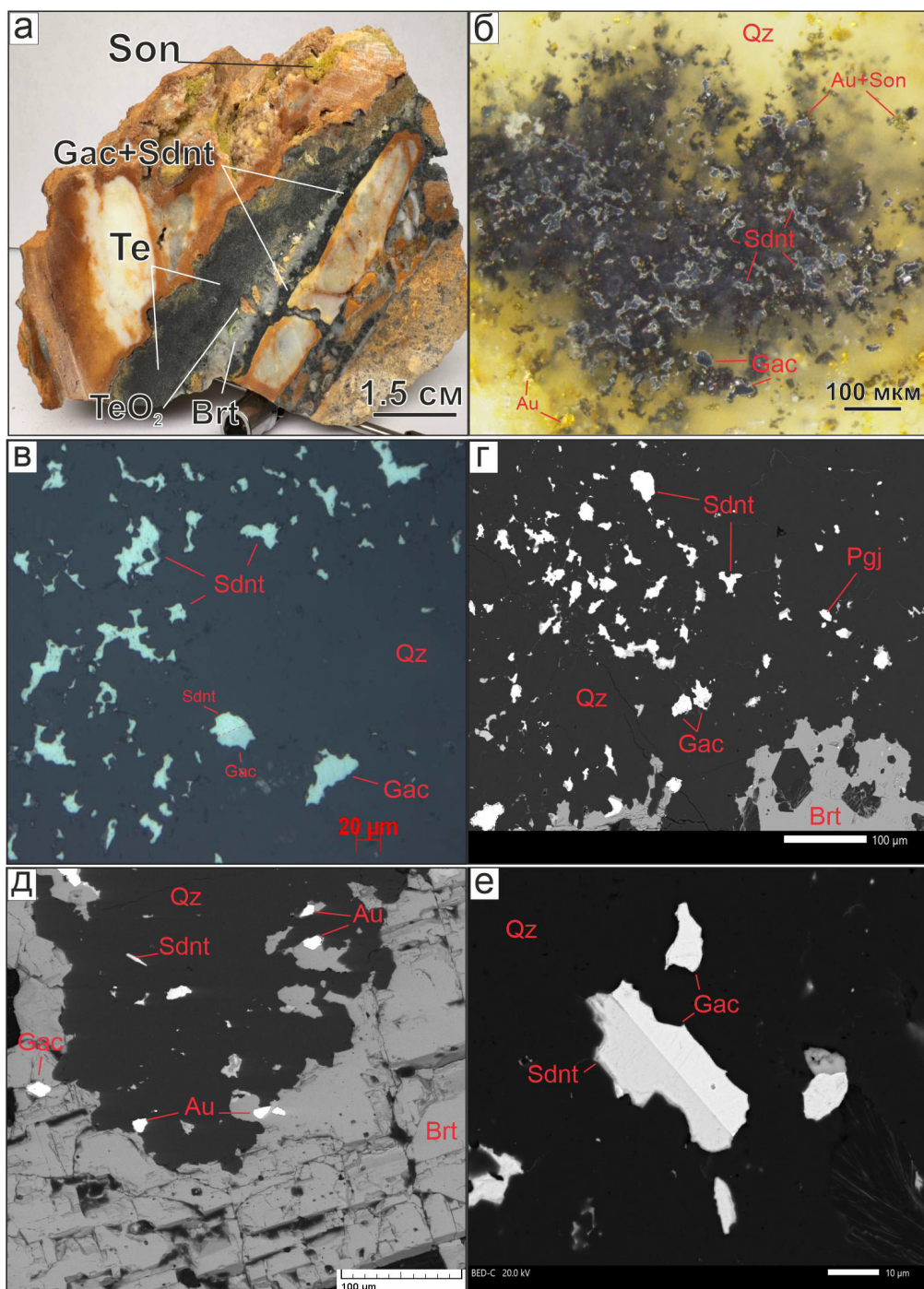
Рис. 1. Минералы золото-гачингит-селенодантопаитовой ассоциации в руде Озерновского месторождения: а – фрагмент богатой самородным теллуrom барит-диксит-кварцевой жилы с кокардово-брекчиевой текстурой в тектонизированном аргиллизите; б, в – обособления гачингита, селенодантопаита и самородного золота в кварце; г – селенодантопаит, гачингит и парагуанахуатит в кварце; д – кварц и барит с включениями гачингита, гипогенного самородного золота и селенодантопаита; е – сросток гачингита и селенодантопаита. Фотография (в) – в отраженном свете; изображения (г), (д) и (е) сделаны под сканирующим электронным микроскопом в режиме обратно-рассеянных электронов (BSE). Au – самородное золото, Brt – барит, Gac – гачингит, Mda – мандариноит, Pgj – парагуанахуатит, Qz – кварц, Te – Se-содержащий самородный теллур, Sdnt – селенодантопаит, Son – сонораит.
