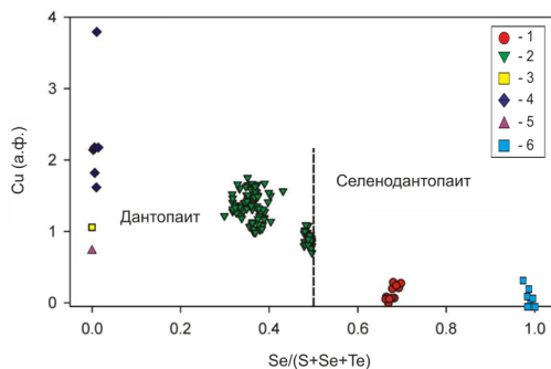
Рис. 4. Соотношение количества примесной Cu (в атомах на формулу, рассчитанную на сумму всех атомов, равную 40) и атомной доли Se в халькогенидной части формулы (S+Se+Te) у минералов ряда дантопаит – селенодантопаит из разных месторождений мира: 1 – Принц Эвжен, Чехия; 2 – Мохавк, Голдфилд, Невада, США; 3 – Эрцвайс, Австрия; 4 – Розалия, Словакия; 5 – Юго-Корневское, Южный Урал [Sejkora et al., 2025, и ссылки в этой работе]; 6 – Озерновское, наши данные.
